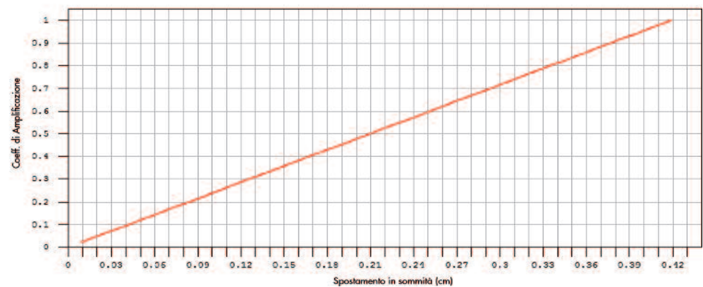
Figura 34 Curva di capacità relativa allo spostamento lungo Y della sommità SW del Palazzo soggetto ad accelerazione crescente da 0 a 0.362 g (accelerazione di progetto per il modo principale secondo la direzione Y).
