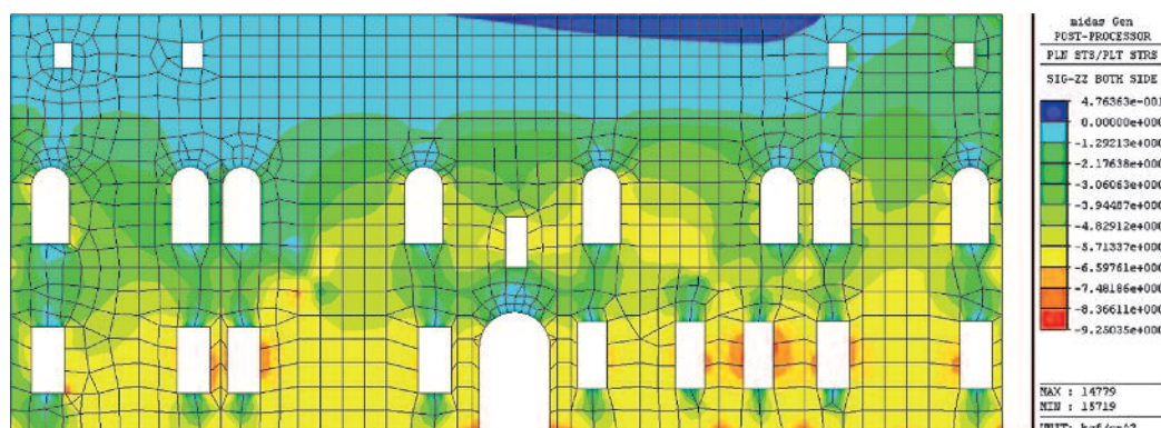
Figura 10 Tensione di compressione alla base: 0.65 \div 0.75 N/mm 2 .
