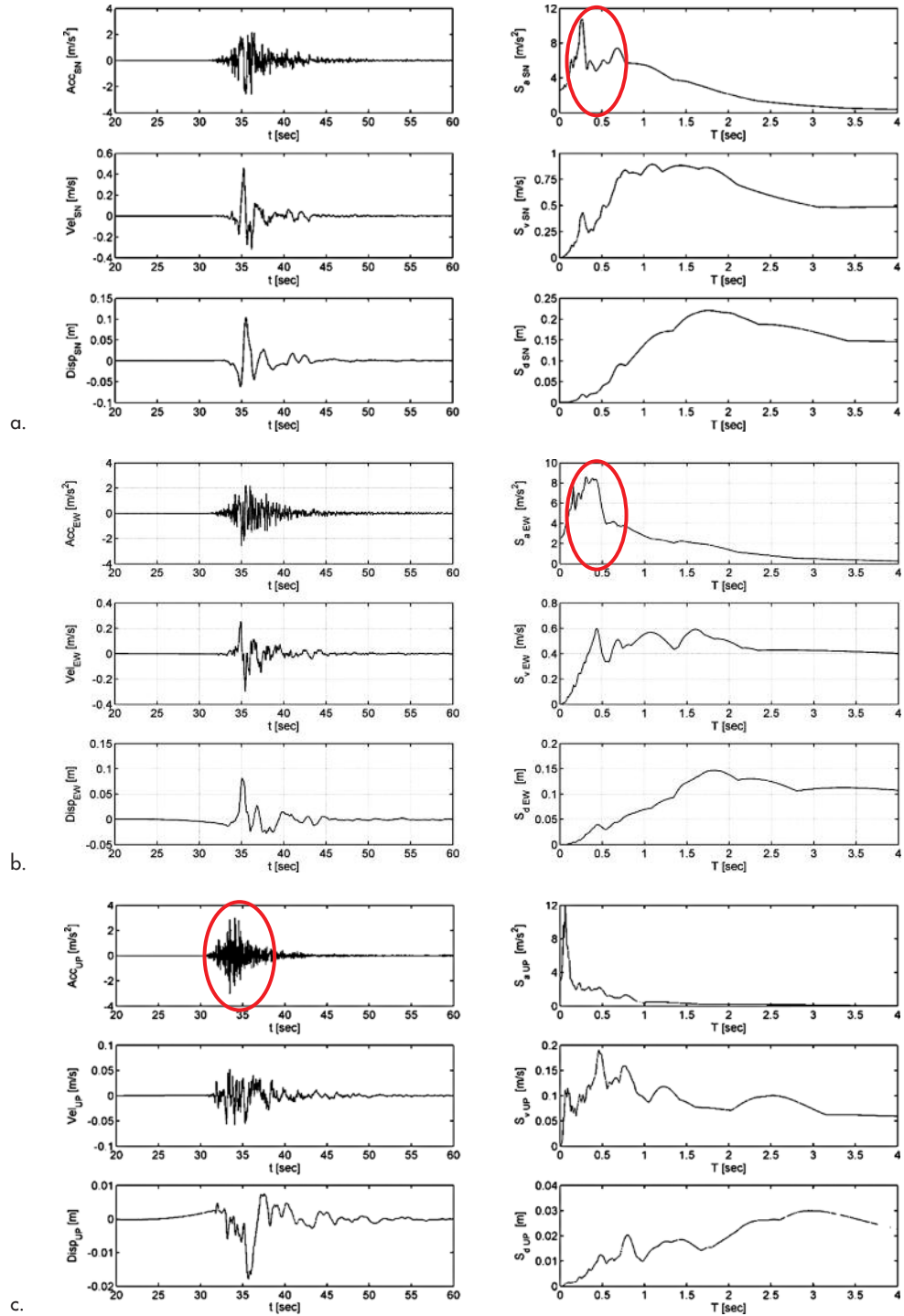
Figura 6 Registrazioni della stazione RAN di Mirandola (MO) dell'evento del 20 maggio ora UTC 2:03:52. Nella colonna di sinistra sono rappresentati gli scuotimenti in termini di accelerazione, di velocità e di spostamento, nella colonna di destra sono raffigurati i corrispondenti spettri: a) componente Est-Ovest; b) componente Nord-Sud; c) componente verticale (fonte: Protezione Civile Italiana tramite www.terremotoemilia.it).
