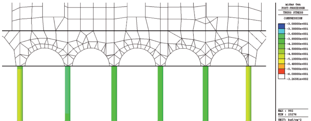
Figura 12 Tensione di compressione alla base: 4.5 \div 5.5 \text{N/mm}^2 .
