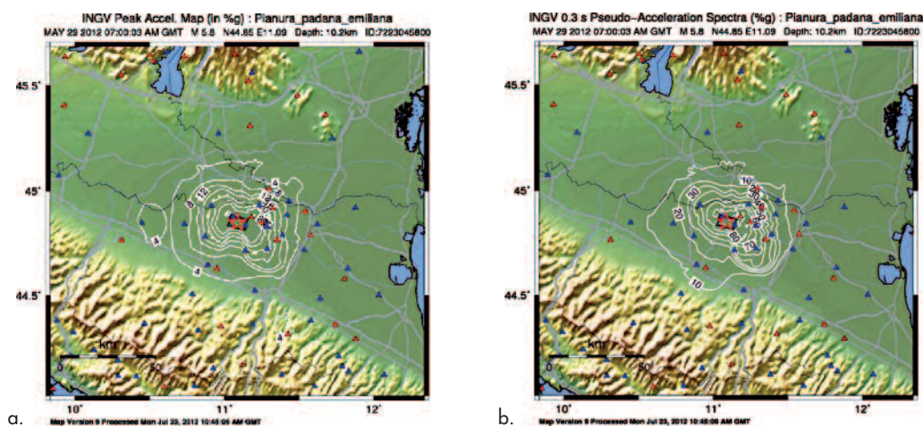
Figura 7 Sisma del 29 maggio 2012, ora UTC 7:00:03: a) l'accelerazione orizzontale al suolo a Correggio risulta prossima a 0.12 g; b) per un periodo di vibrazione di 0.3 s, l'accelerazione è prossima a 0.3 g.
