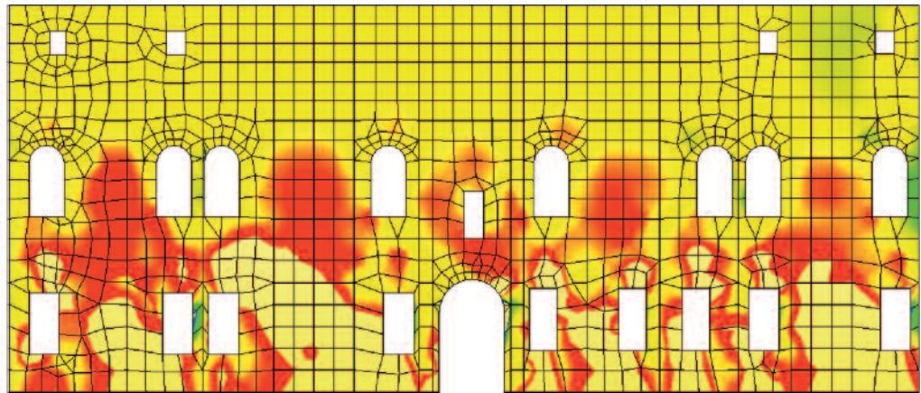
Figura 33 Allineamento A: mappa delle tensioni tangenziali per un'accelerazione pari a 0.8 g (valori di sollecitazione tagliati a \tau = 0.35 \text{ N/mm}^2 ).
