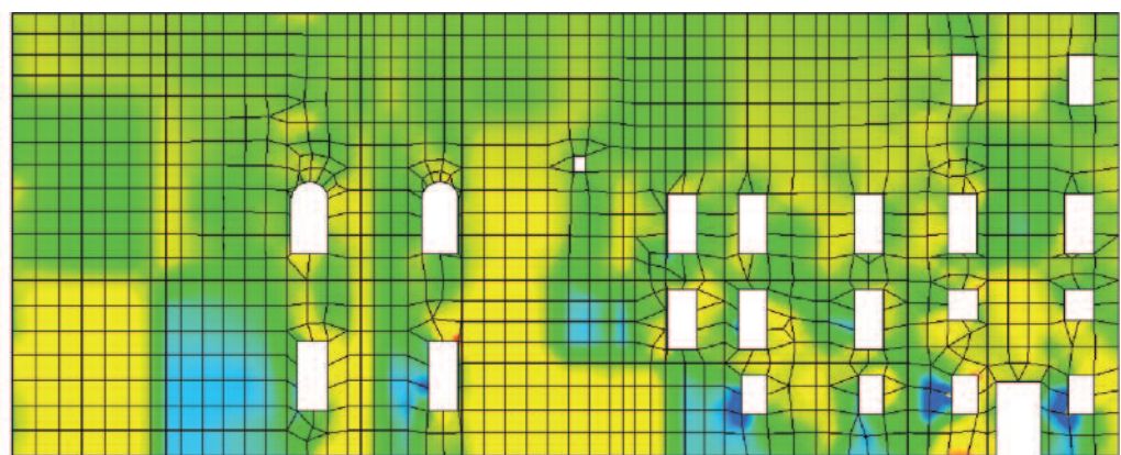
Figura 35 Allineamento 8 Mappa delle tensioni tangenziali per un'accelerazione pari a 0.362 g (valori di sollecitazione tagliati a \tau = 0.35 \text{ N/mm}^2 ).
