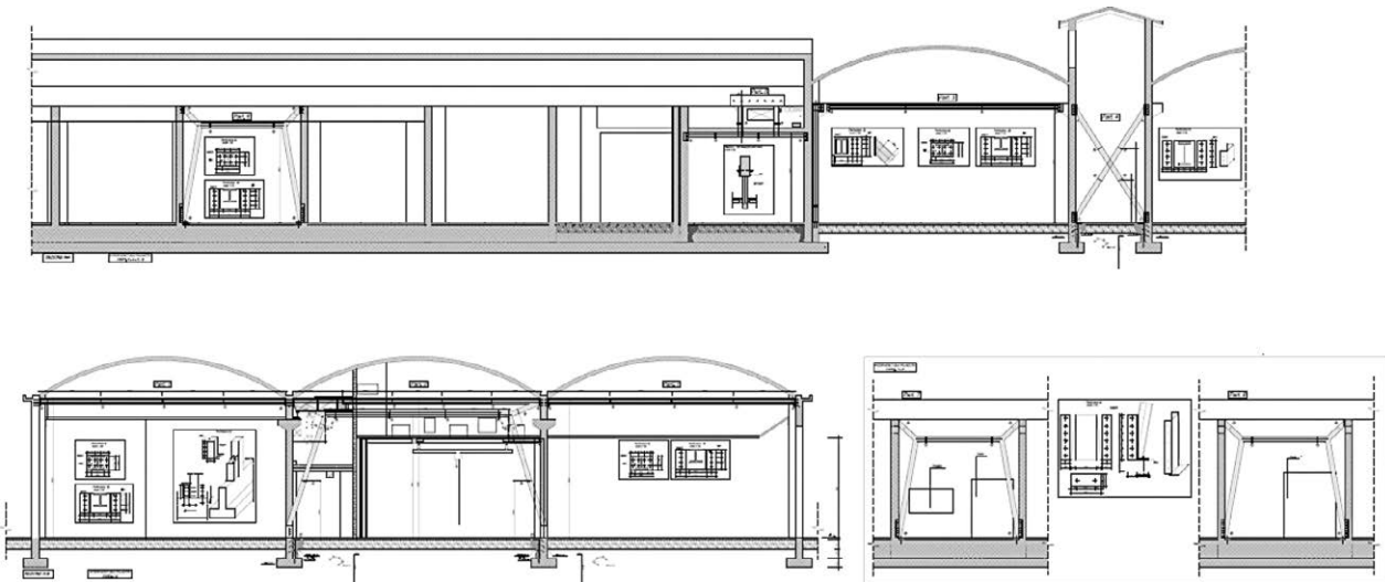
Figura 8 Sezioni tipo dei fabbricati con inserimento degli interventi di miglioramento sismico.
