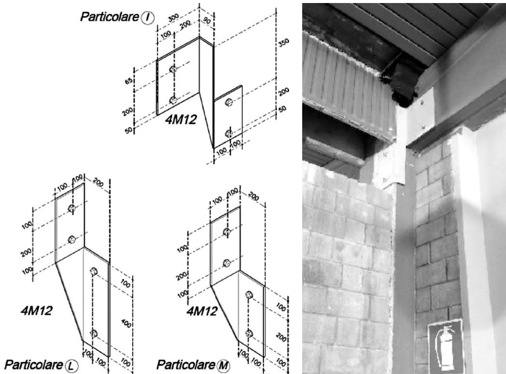
Figura 5 Connessioni tra gli elementi prefabbricati.
