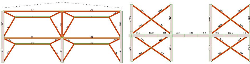
Figura 7 Schemi dei controventi metallici (azioni assiali in KN).
