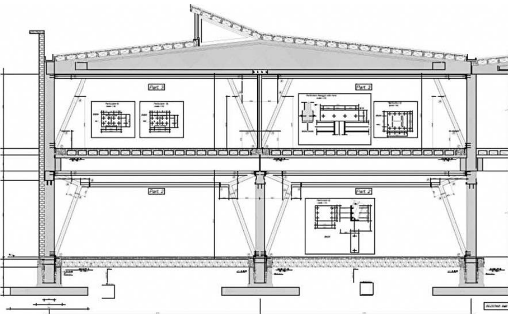
Figura 8 Sezioni tipo dei fabbricati con inserimento degli interventi di miglioramento sismico.
